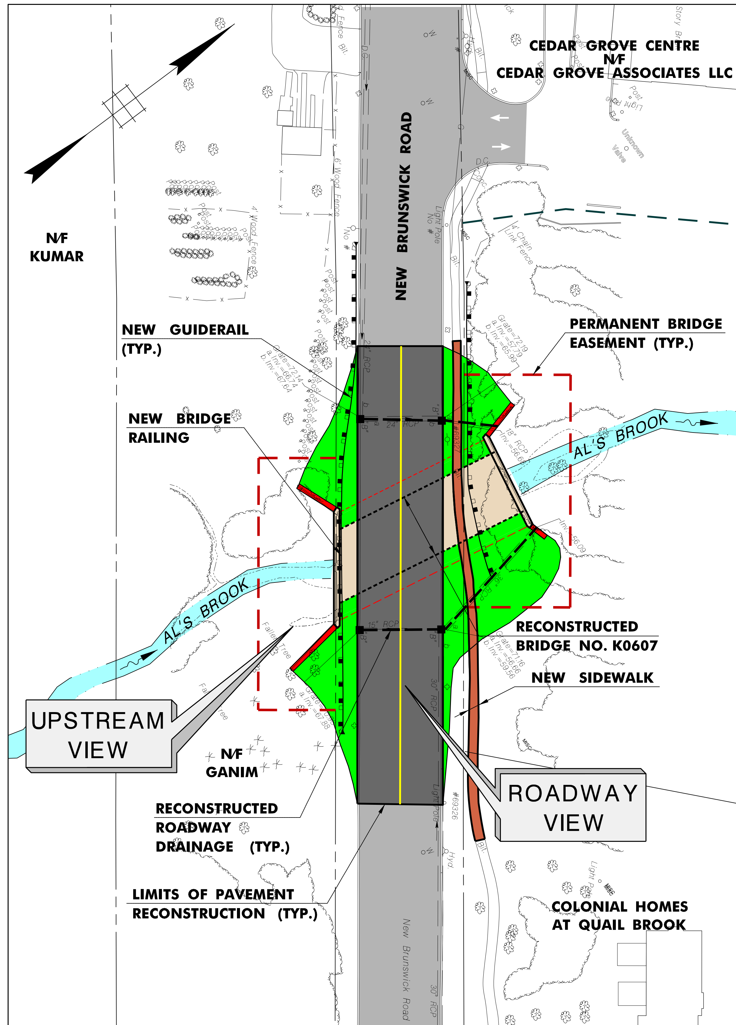
PLAN SCALE: 1"=30'
